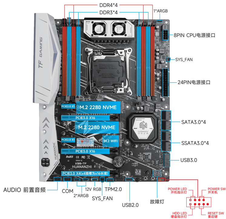
图1-1 X99-TF主板图解
